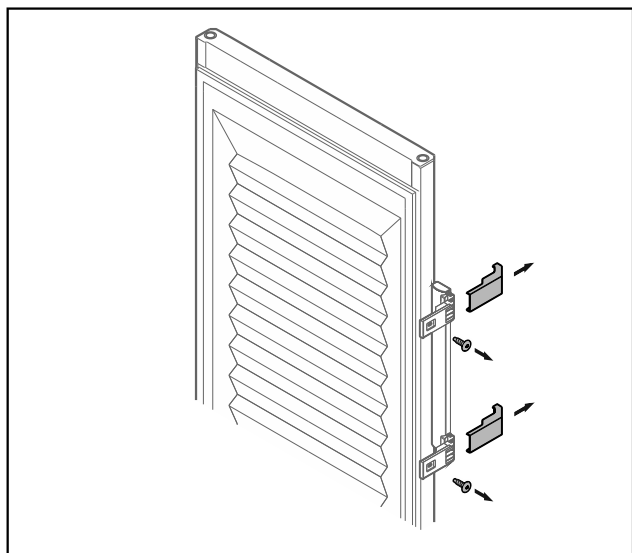
Fig. 26 Drzwi piankowe
