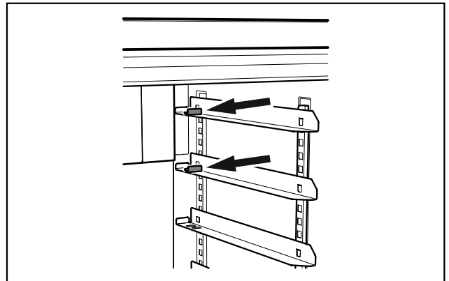
Fig. 55 Wspornik ograniczający
