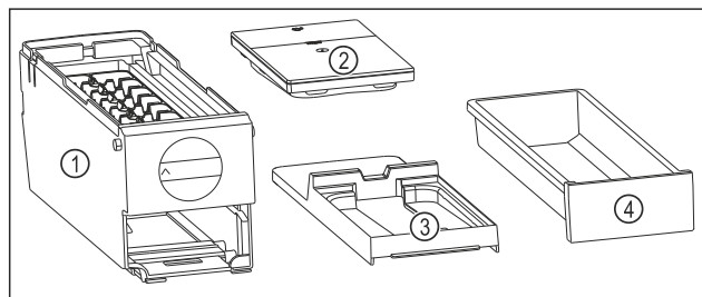
Fig. 81 Sastavni dijelovi sustava EasyTwist-Ice
