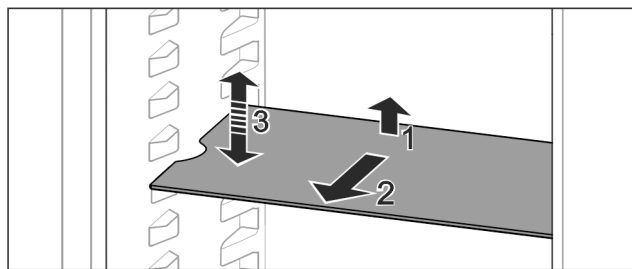
Fig. 126 ▶ 抬起搁板并向前拉出。 ▷ 使侧面凹口位于支撑位置。 ▶ 安装搁板：升降到任意高度并推入。
