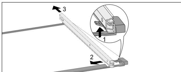
Fig. 48 Tablette en verre avec rails
