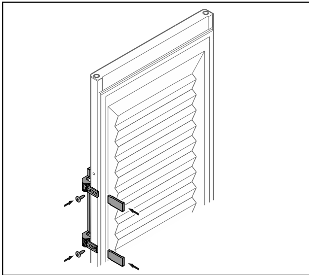
Fig. 32 Skumfylt dør
