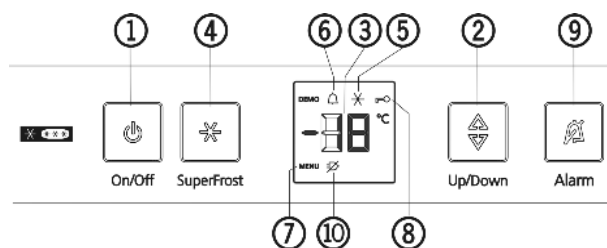
Fig. 3 (1) Бутон On/Off (6) Символ Аларма (2) Бутон за настройка (7) Символ меню (3) Температурен индикатор (8) Символ Защита от деца (4) Бутон SuperFrost (9) Бутон Аларма (5) Символ SuperFrost (10) Символ спиране на тока
