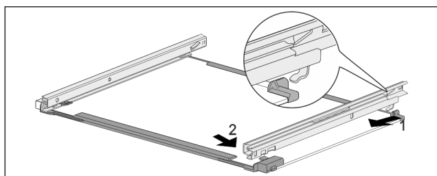
Fig. 119 Stiklinė lentynėlė su bėgeliais
