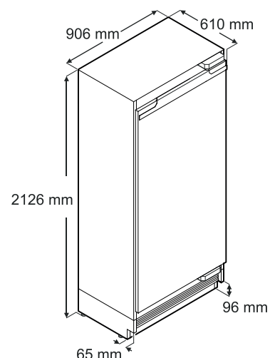
EKB 96.. / ERB.. 99..
