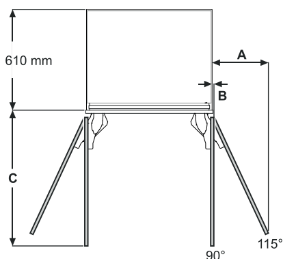
EKB 94.. / ERB.. 97..
