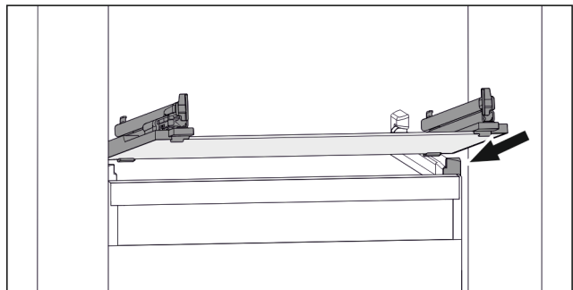
Fig. 167 Lasihyllyn esimerkinomainen kuvaus
