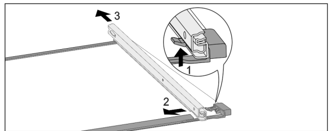
Fig. 190 Lasihylly kiskoilla
