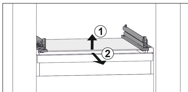
Fig. 98 Ενδεικτική απεικόνιση του γυάλινου ραφιού
