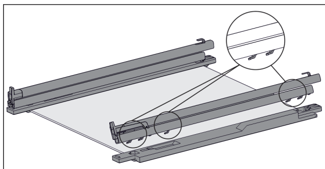
Fig. 150 Tablette en verre avec rails et pièces de retenue
