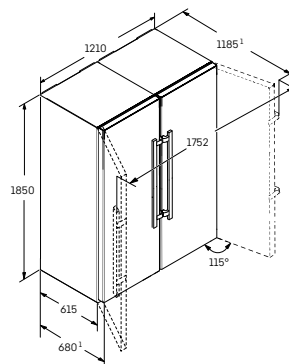
尺寸图：
