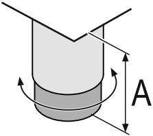
Fig. 12 Podesivu nožicu moguće je namjestiti od A = 115 \text{ mm} (4 1/2 in) do 175 \text{ mm} (6 7/8 in).
