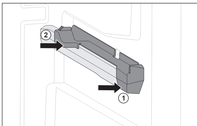
Fig. 63 Tillsats på den högra behållarens galler
