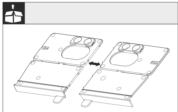
Fig. 23 Montagewinkel Boden
