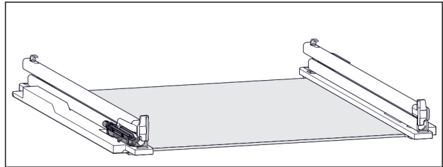
Fig. 99 Unitate de amortizare
