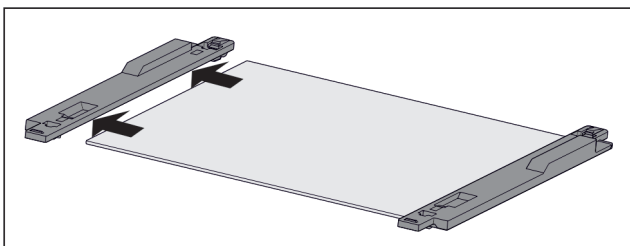
Fig. 97 Placă de sticlă cu piese de fixare
