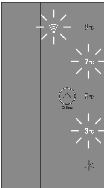
Fig. 46 Ένδειξη σε περίπτωση σφάλματος WLAN
